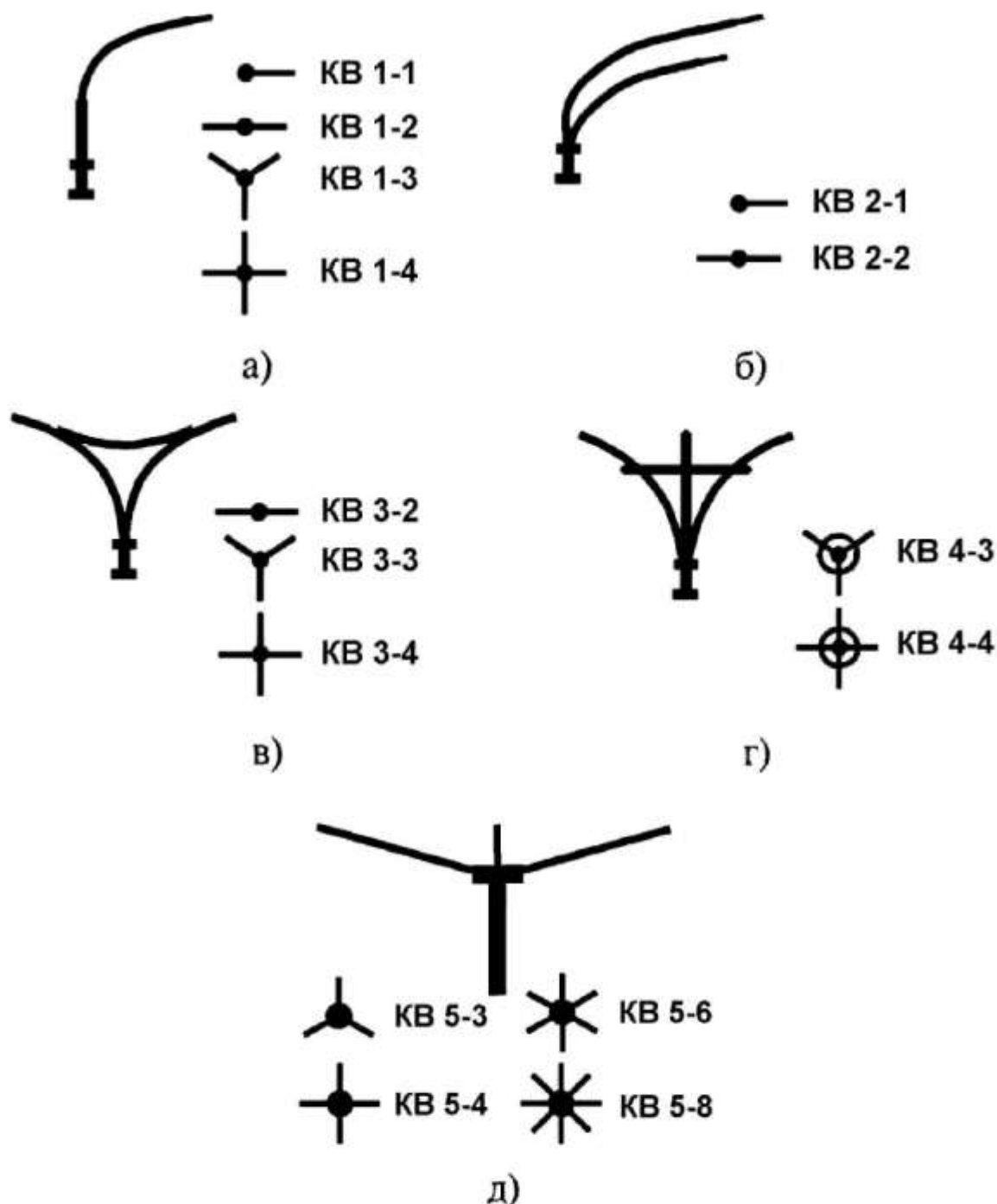
Рис. 4.2. Варианты верхних кронштейнов к ОКС-1 а) KB 1; б) KB 2; в) KB 3; г) KB 4; д) KB 5
